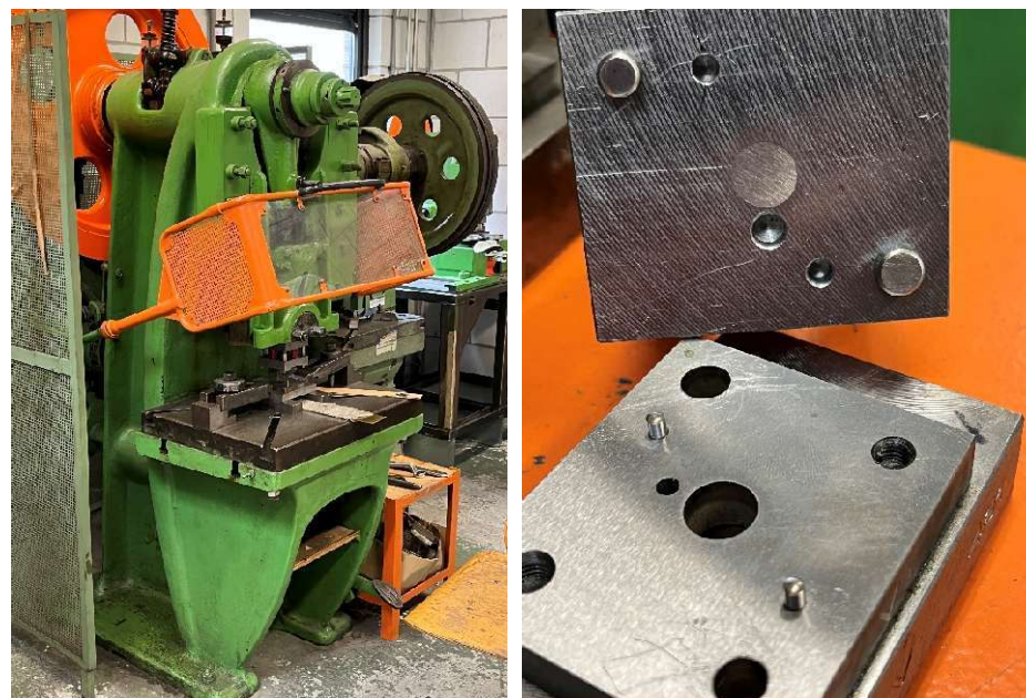
Links de excenterpers, rechts de feitelijke stans
